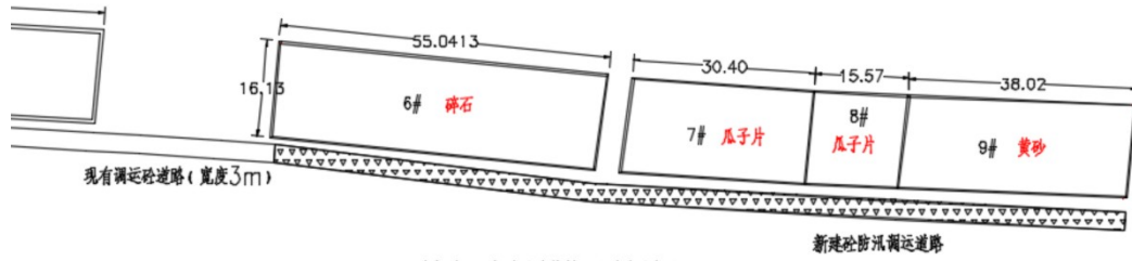
上桥管理所拆除重建物料池及道路示意图
