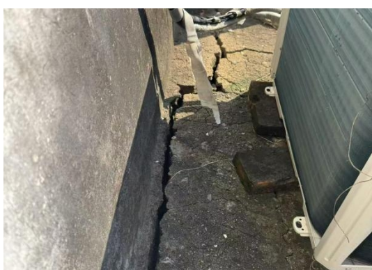
散水损毁、不均匀沉降
