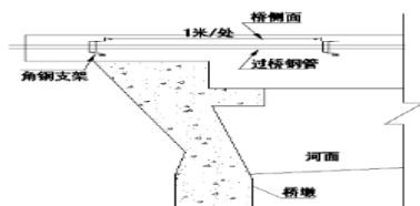
图 过桥、涵闸口方式一
