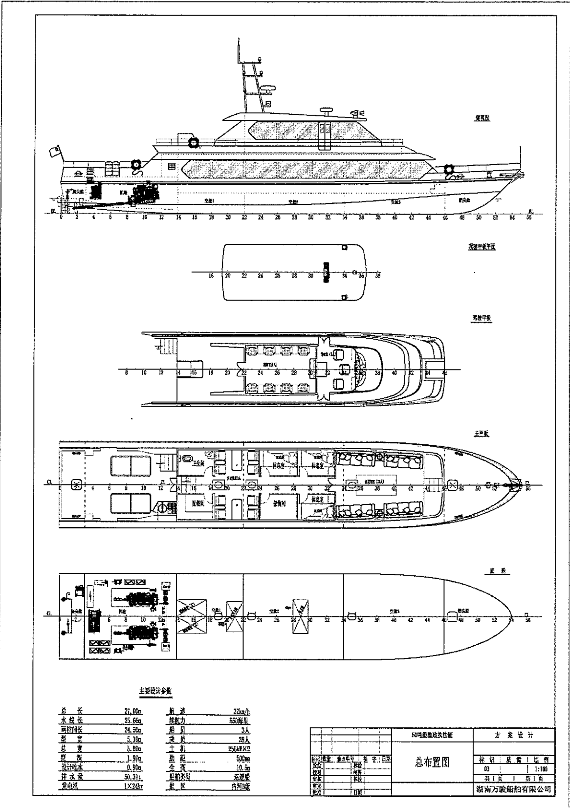
附件 2: 50 吨级渔政执法船总布置图
