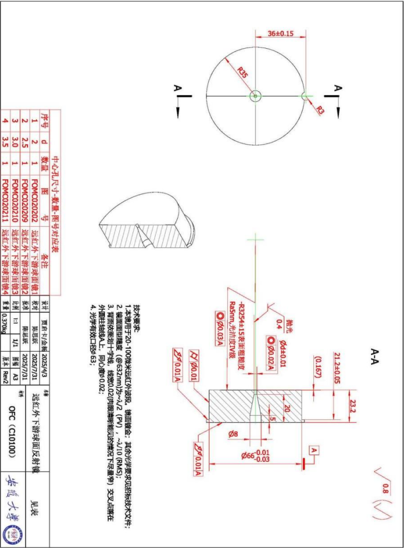
图 4 远红外下游球面镜
