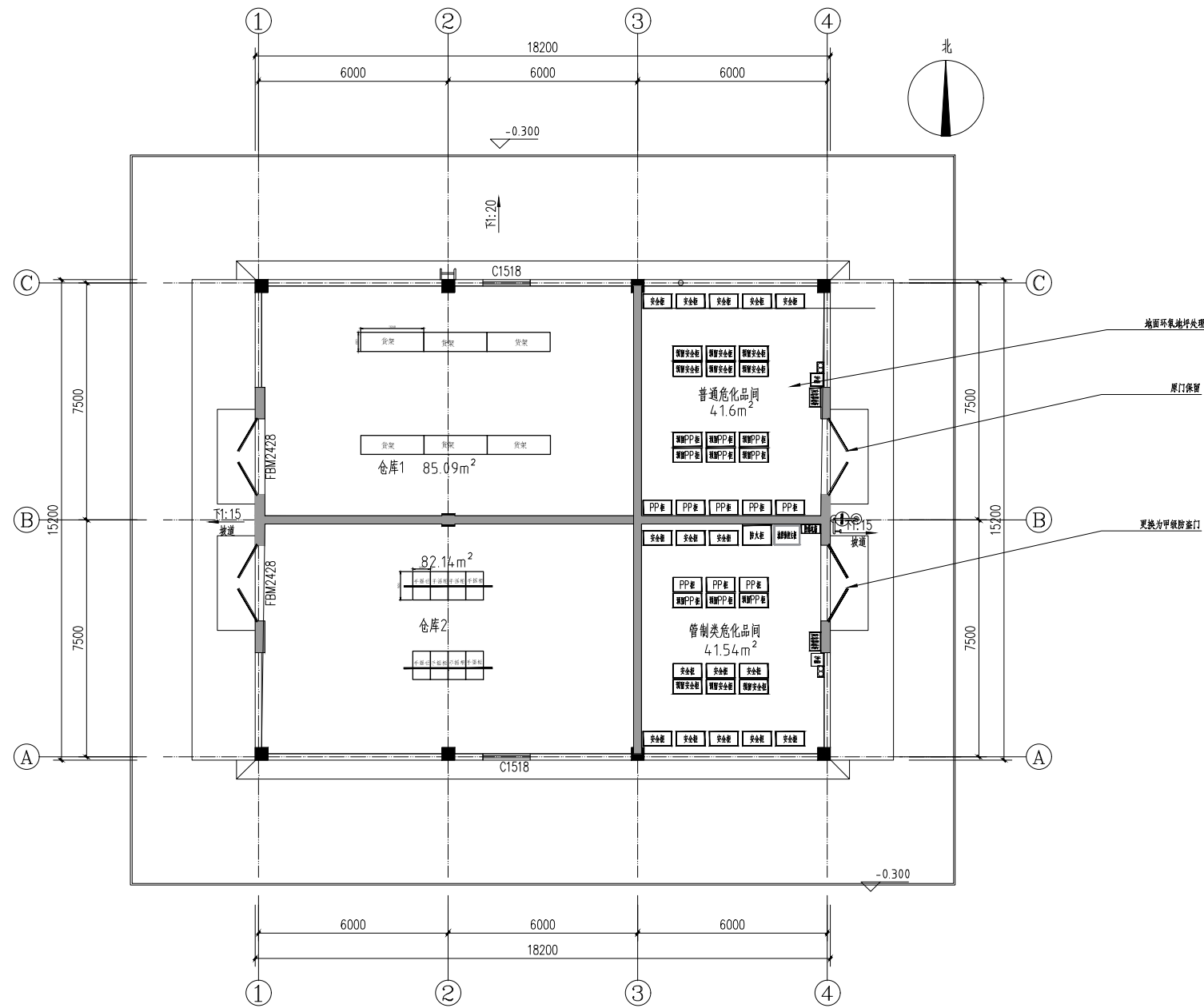
工艺布置图 1:150
