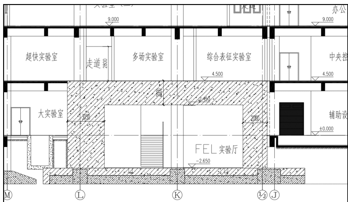
图 2 FEL 大厅的剖面图和顶棚厚度
